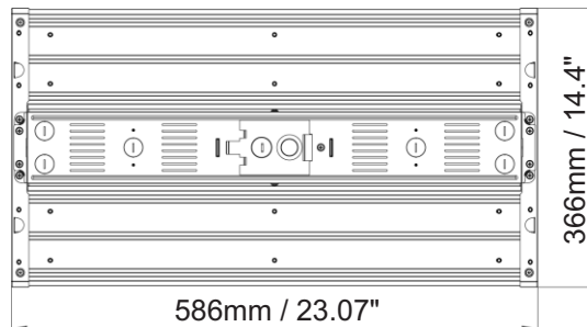
PHBF - 105W & 165W Dimensions mm | 586(L) x 366(W) x 48(D) inch | 23.1(L) x 14.4(W) x 1.9(D)
