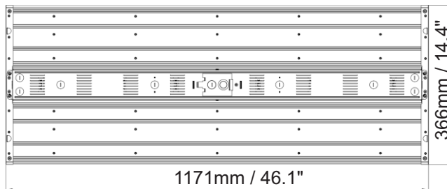
PHBF - 225W & 300W Dimensions mm | 1171(L) x 366(W) x 48(D) inch | 46.1(L) x 14.4(W) x 1.9(D)
